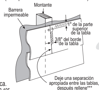
TRATAMIENTO DE JUNTAS – OPCIÓN 2 (No aplica al acabado ColorPlus®)
