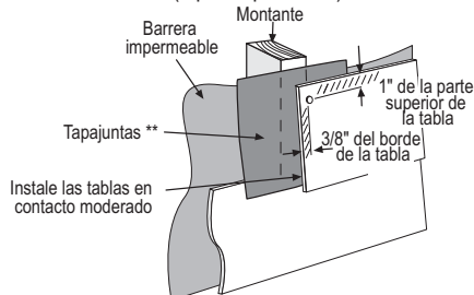
TRATAMIENTO DE JUNTAS – OPCIÓN 1 (Opción preferida)
